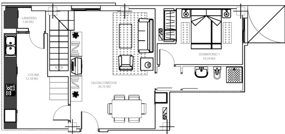
PLANTA 5ª
